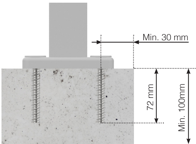
SCHRAUBE FÜR BETONBEFESTIGUNG
